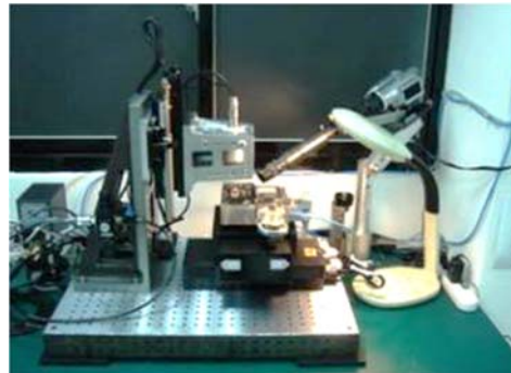
微型CNC複合工具機
