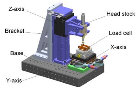
智能化玻璃鑽孔機
